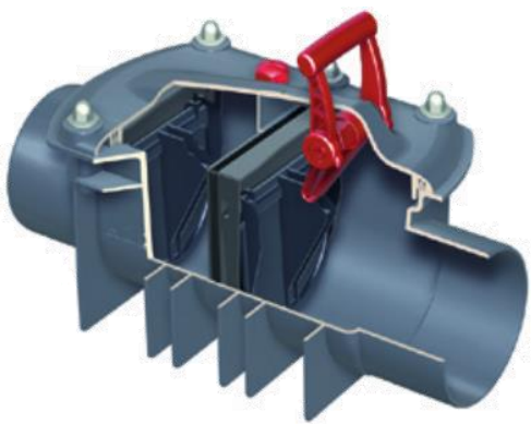
Rückstausicherung im Gebäude für nicht fäkalienhaltiges Abwasser
